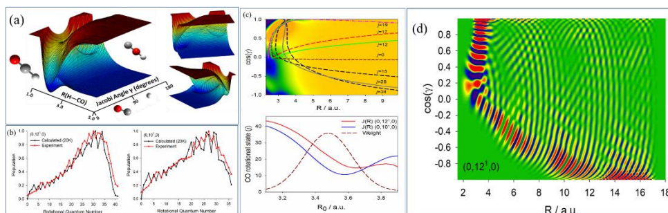
(a) HCO 基态与 A 态势能面示意图 (b) 实验测量与理论模拟产物转动态分布
